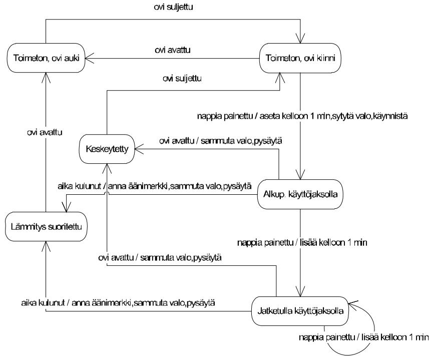
Kuva 5.51: Mikroaaltouuni. Alkutilassa mikroouuni on toimeton ja ovi on kiinni. Oven avaamisen jälkeen uuni pysyy edelleen toimettomana. Mikro käynnistetään nap- pia painamalla (oven pitää olla kiinni), jolloin mikroon syttyy valo ja asetetaan mi- nuutin käyttöaika. Aikaa saadaan minuutti lisää jokaisella uudella painalluksella. Jos ovi avataan kun aikaa on vielä jäljellä, lämmitys keskeytetään, valo sammutetaan ja aika nollataan. Mikroouuni palaa toimettomaksi, kun ovi suljetaan. Normaalitypauk- sessa ajan annetaan kulua loppuun, jonka jälkeen mikroouuni antaa äänimerkin, uuni pysäytetään ja valo sammutetaan. Kun ovi avataan, mikroouuni palaa toimettomaksi.
