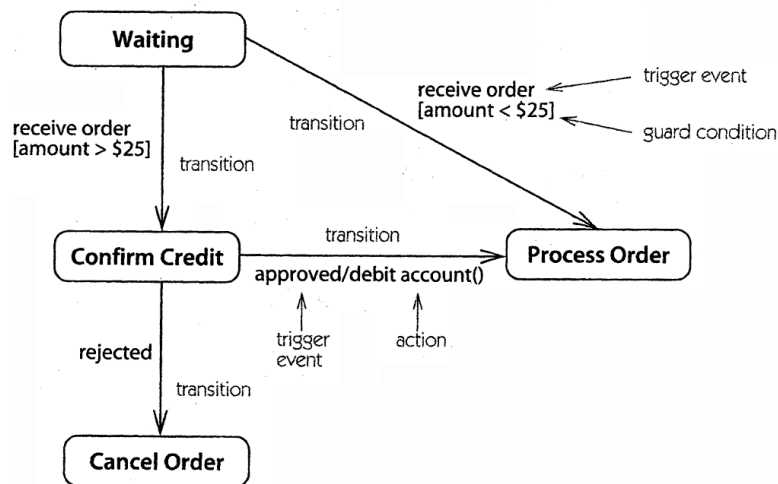
Kuva 5.47: Tilakaavio tilauksen käsittelylle. Tilauksen käsittelyjärjestelmä odottaa tilausta. Kun tilaus otetaan vastaan, se käsittelee tilauksen, mikäli tilauksen arvo on alle 25 dollaria. Yli 25 dollarin tilauksissa se varmistaa ensin luoton. Mikäli luottoa on tarpeeksi, se käsittelee tilauksen. Muussa tapauksessa se peruuttaa tilauksen.
