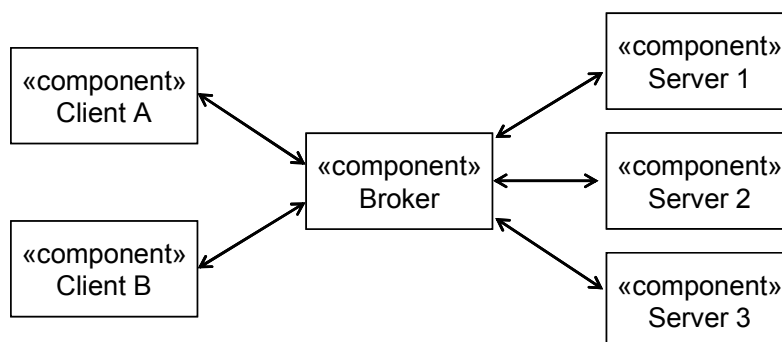
Kuva 5.21: Välittäjä-arkkitehtuurimalli
