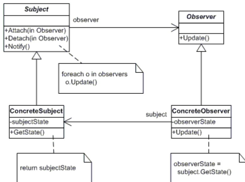
Kuva 5.26: Tarkkailija-malli
