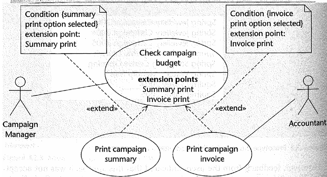
Kuva 3.5: Mainostoimistoesimerkin (Bennett 2006) käyttötapaus ”tarkasta kampanja-budjetti” lyhennelmänä, 2-sarakemuodossa ja käyttötapauskaavion osana. Huom. käyttötapauksen vaiheiden kuvauskäytännössä on pieniä ongelmia: ”none”-niminen vaihe ja yleinen ”Actor”-niminen rooli.
