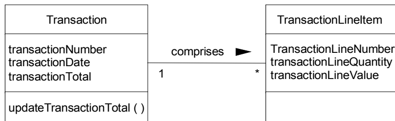
Kuva 5.22: Transaction-Transaction Line Item -analyysimallin esitys luokkakaaviona
