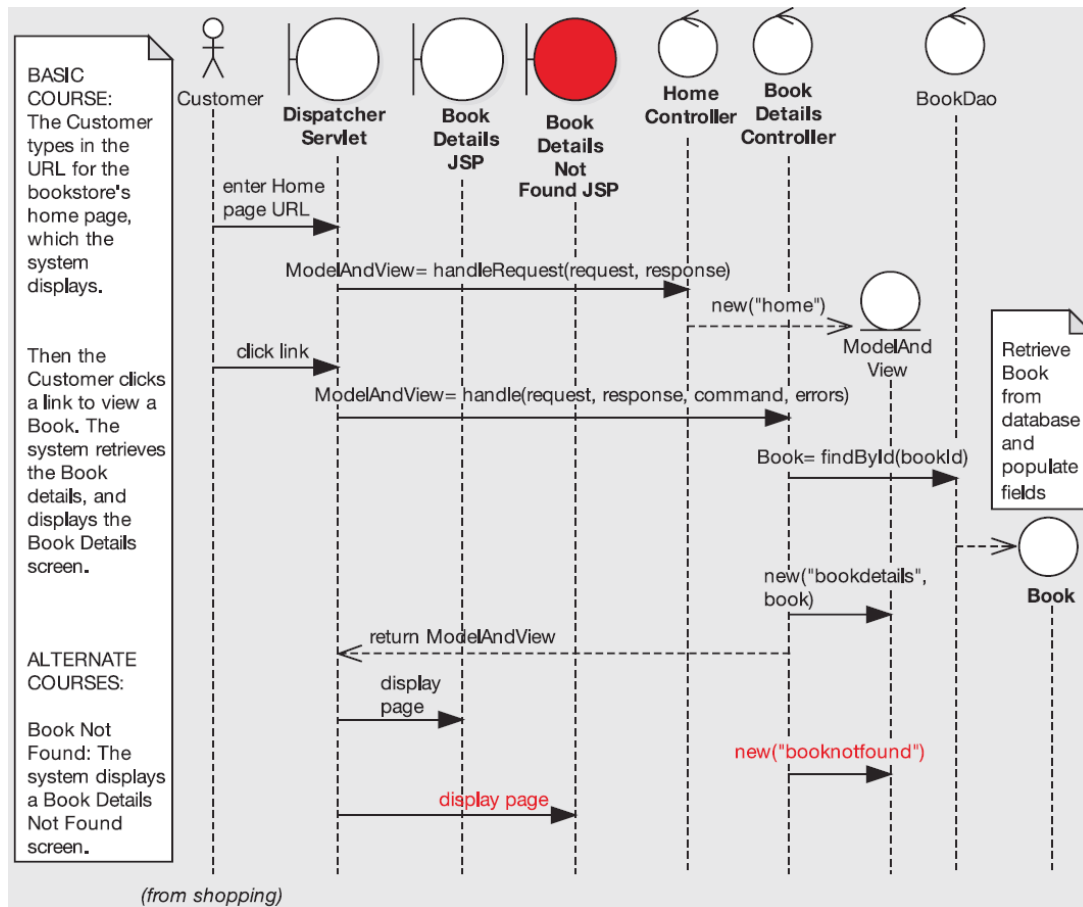
Kuva 4.32: "Näytä kirjan tiedot"-käyttötapauksen sekvenssikaavio.
