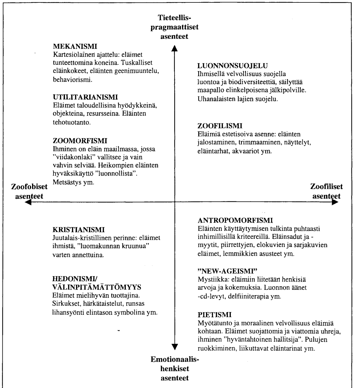
KUVIO 3. Länsimaisen kulttuurin ihmiskeskeiset suhtautumistavat eläimiin (Martinelli 2002).
