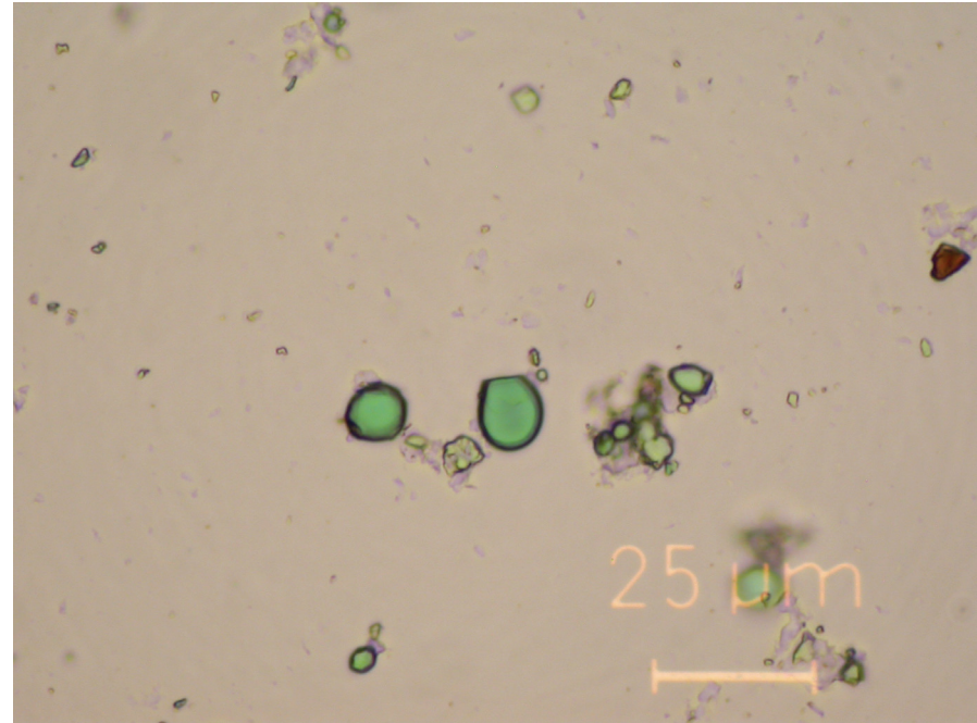
Kuva 7. Koboltinvihreä-väriainepartikkeleita tasopolarisoidussa läpivalossa. Näyte teoksesta Aallottaria , 1909. Öljyväri kankaalle, 53,5 x 73 cm. Ateneum, Helsinki. Kansallisgalleria, inventaarionumero A-1995-96. Kuva: Kansallisgallerian materiaalitutkimuslaboratorio / Seppo Hornytzkyj. (Linkki teoskuvaan: https://www.kansallisgalleria.fi/fi/object/501754 ).
