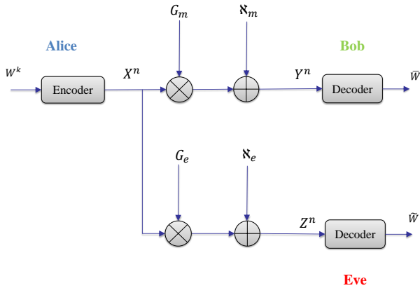
Fig. 1: Fundamental wiretap scenario.
