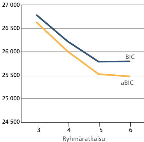
Kuvio 2. Ryhmämerkitysten 3–6 tarkastelu elbow plotin avulla.
