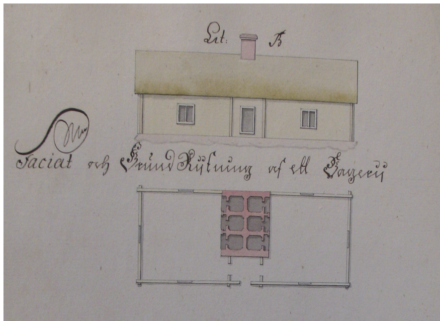
KUVA 2 Julkisivu- ja pohjakuva Lappeenrannan varuskunnan käyttöön suunnitellusta kuusiuunisesta leipomosta
