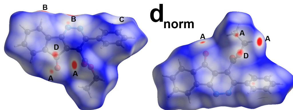
Figure 12. The d_{\text{norm}} Hirshfeld surfaces of 10 : (A) O...H, (B) N...H, (C) C...O, (D) C...H.
