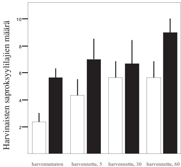
Kuva 2. Harvinaisten saproksyyililajien määrät koaloilla. Mustat pylväät kuvaavat poltettuja aloja ja valkeat pylväät polttamattomia. X-akselilla on kuvattu hakkuukäsittely ja tuotetun lahpuun määrä ( m^3 / ha ).
