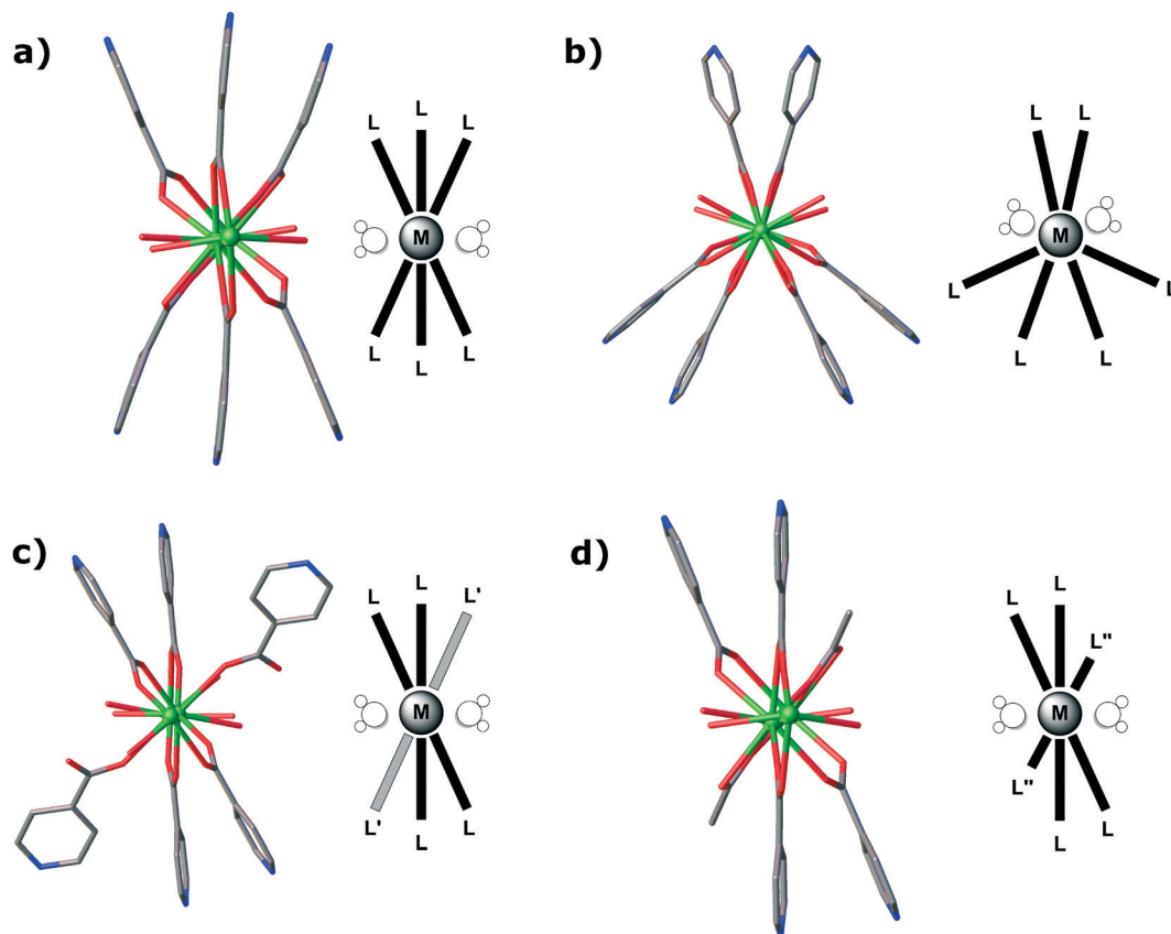
Fig. 10 Ligand orientations of a) TTPPC \text{NdBr}_3 , b) TTPPC \text{NdBr}(\text{OTf})_2 , c) TTPPC \text{Nd}(\text{OTf})_3 and d) TTPPC \text{NdBr}_2\text{OAc} along the water channel direction (hydrogen atoms omitted for clarity).
