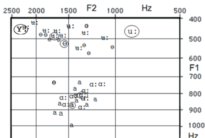
Figur 3. f1 och f2 hos T2 i betonade [a] (n=9), [ɑ:] (n=9), [e] (n=9) och [ɥ:] (n=9) i det första testet. De inringade symbolerna ger f1-f2-medelvärde för [y:], [ɥ:], [e], [u:], [ɑ:] och [a] (minst 6 uttal per vokal per medelvärde).
